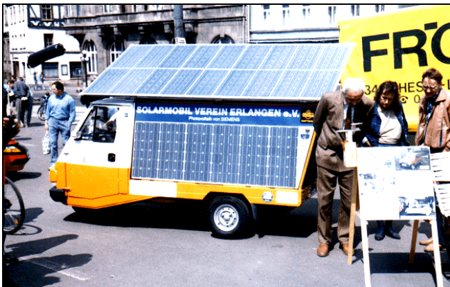
Vespa Piaggio Mobil, Kleinlieferwagen, 600 Watt solar
