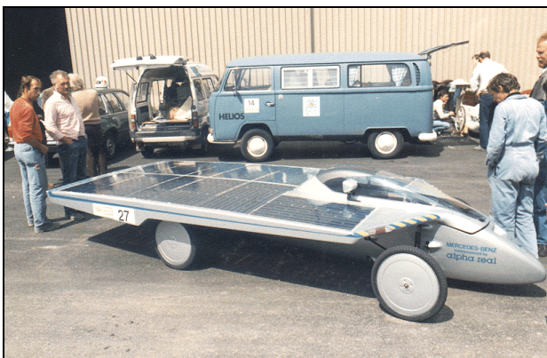
Autarkes Rennfahrzeug Mercedes Solarrennen, Tour de Sol 1985
